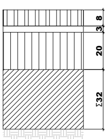
TRINKELIŲ DANGOS ĮRENGIMO ĮRENGIMO DETALĖ D-1
